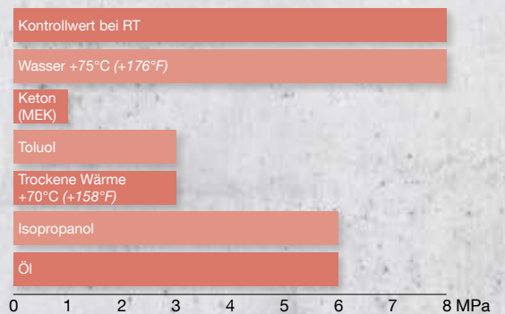
Alterungsbeständigkeit von PP-Verklebungen nach Einlagerung in verschiedenen Medien (14 Tage bei Raumtemperatur)
