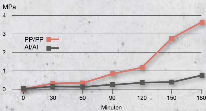
Festigkeitsentwicklungen von WEICON Easy-Mix PE-PP 45 an Zugscherproben nach DIN EN 1465
