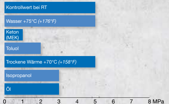
Alterungsbeständigkeit von PE-Verklebungen nach Einlagerung in verschiedenen Medien (14 Tage bei Raumtemperatur)
