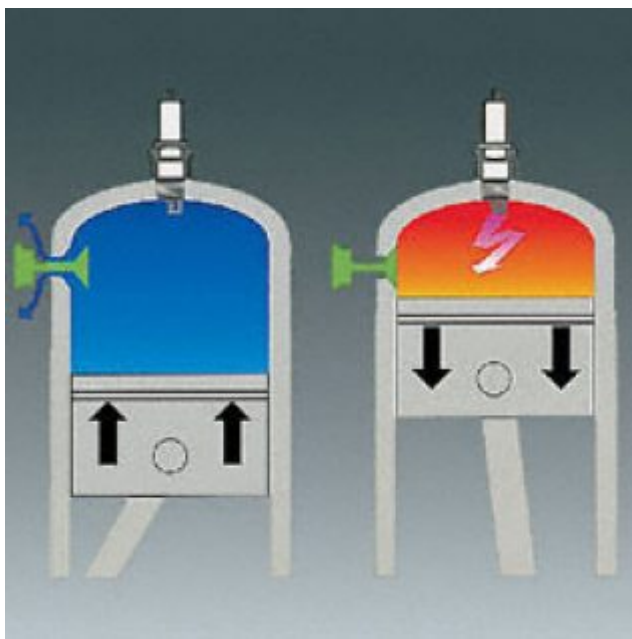
DEKOMPRESIJSKI VENTIL
